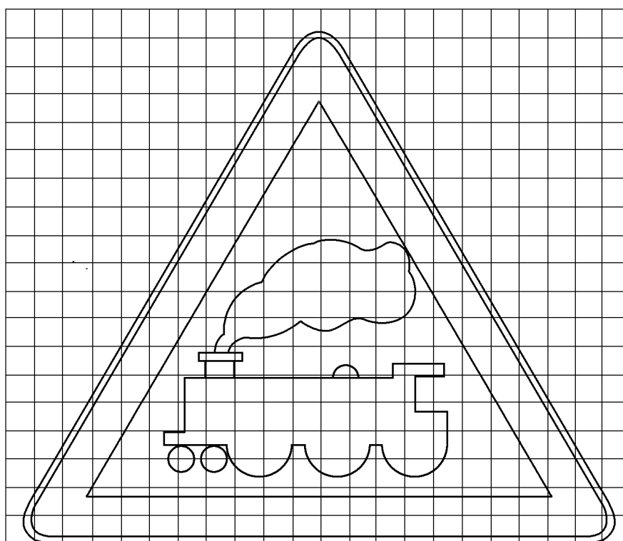
图 4 铁路道口标志版面制作示例图
