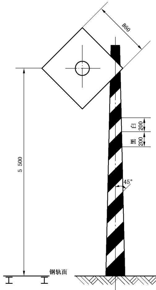
图 2 遮断信号机
