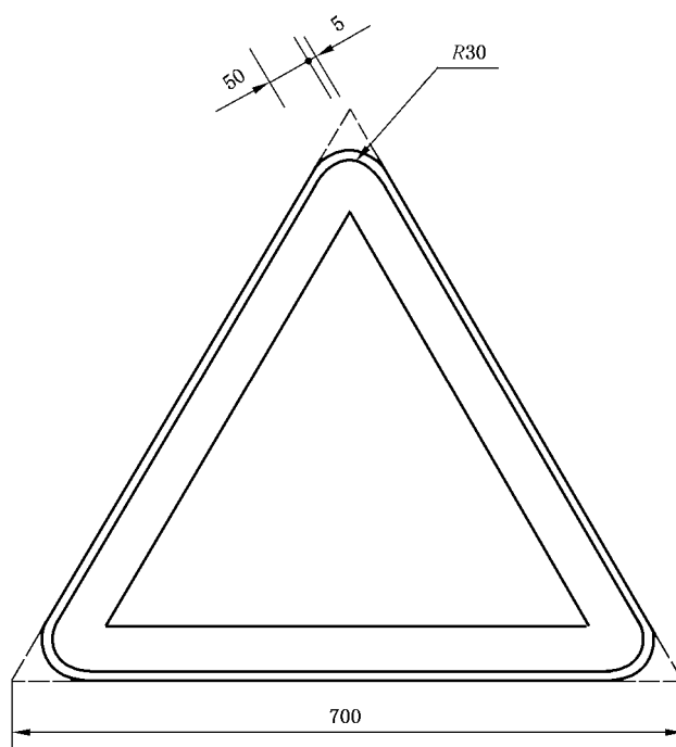
图 3 标志版面尺寸图
